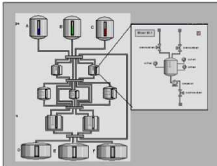
Figur 1 En batchanläggning.
