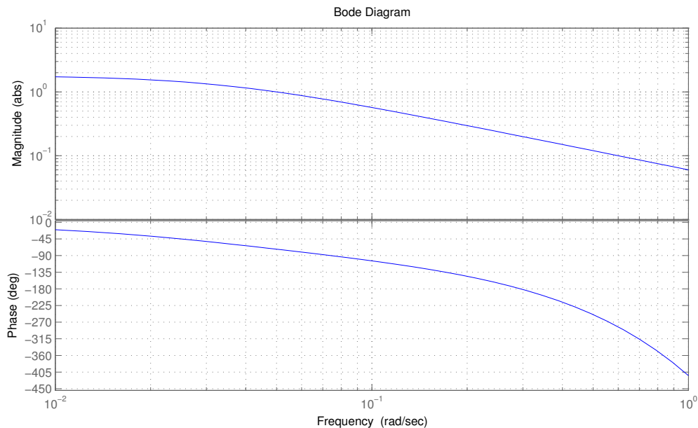
Figure 6.4 Bodediagram i uppgift 6.7
